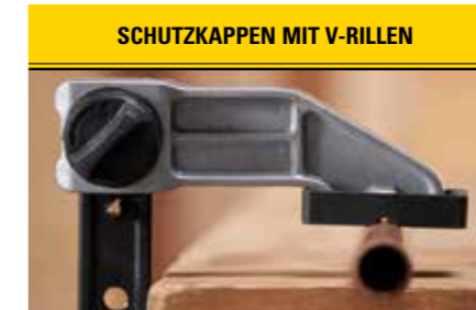
SCHUTZKAPPEN MIT V-RILLEN Effektives Einspannen von zylindrischen oder unregelmäßig geformten Werkstücken wie z. B. Rohre.
